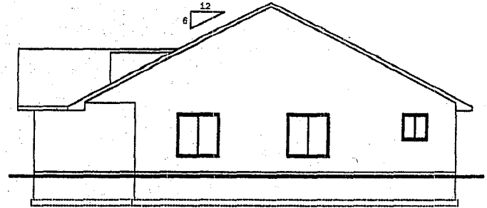
RIGHT ELEVATION
